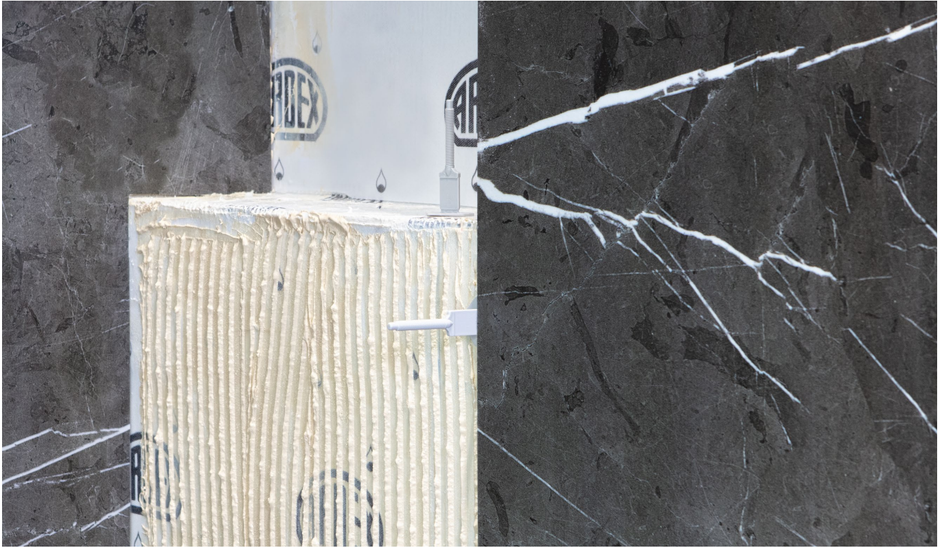
Gewindelaschen für 2 mm Fuge
